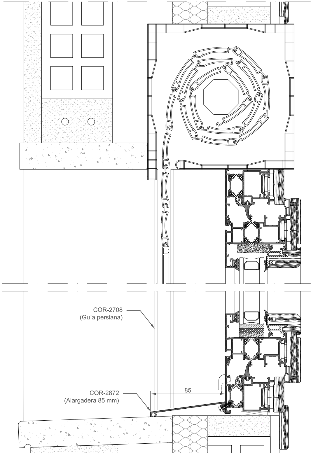
SECCIÓN VERTICAL (B-B)
